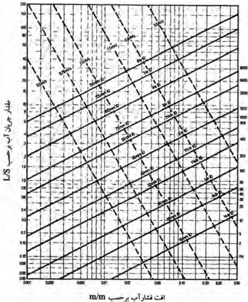
شکل پ - ۱ - ۵ - ۴ ت (SI) منحنی اندازه‌گذاری لوله‌های فولادی گالوانیزه
